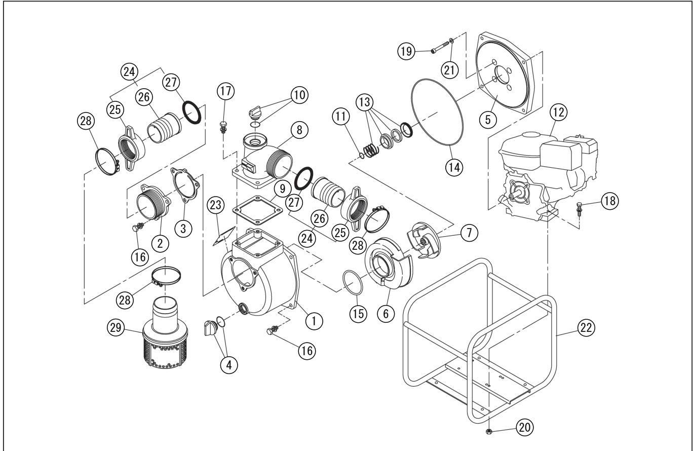
DWG No.070851305 MODEL : SEH-80X FORM : SEH-80X-BFB-0
